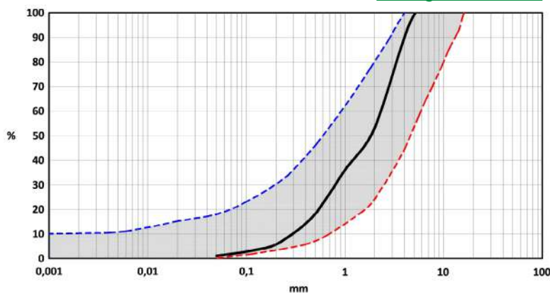
Curva granulometrica
