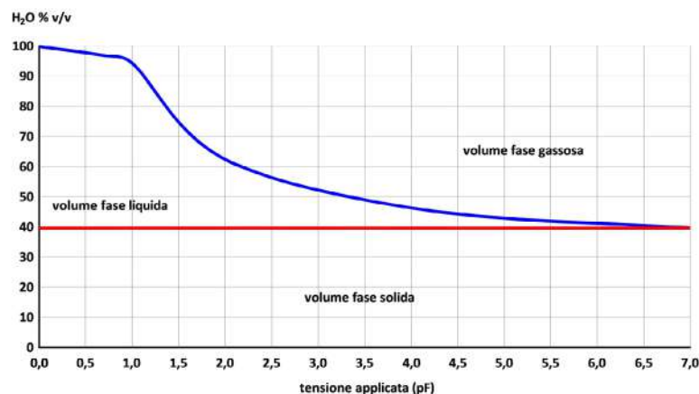
Curva ritenzione idrica
